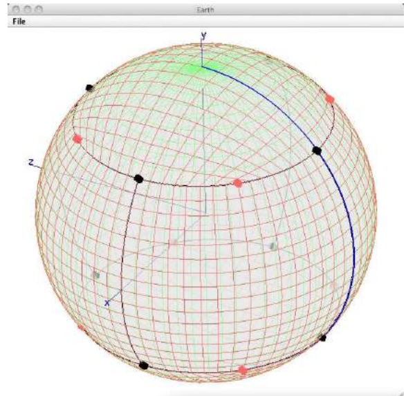
Fig. 5(d): Fourth level of subdivision
